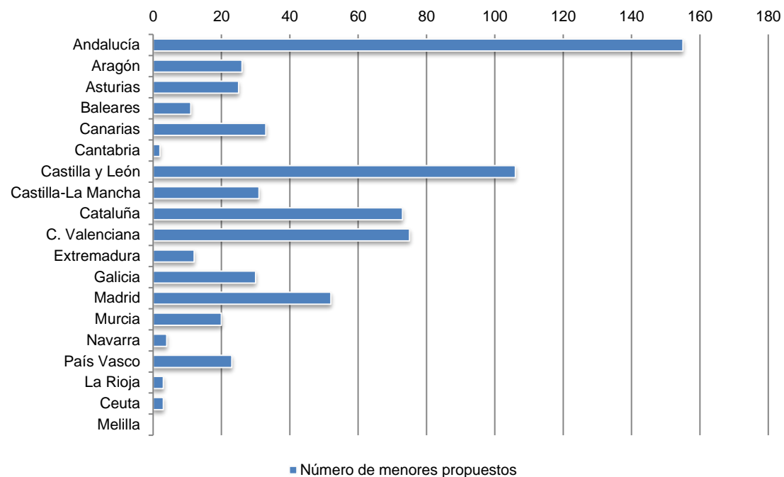
Gráfico 66. Adopción nacional - Número de menores de edad propuestos
